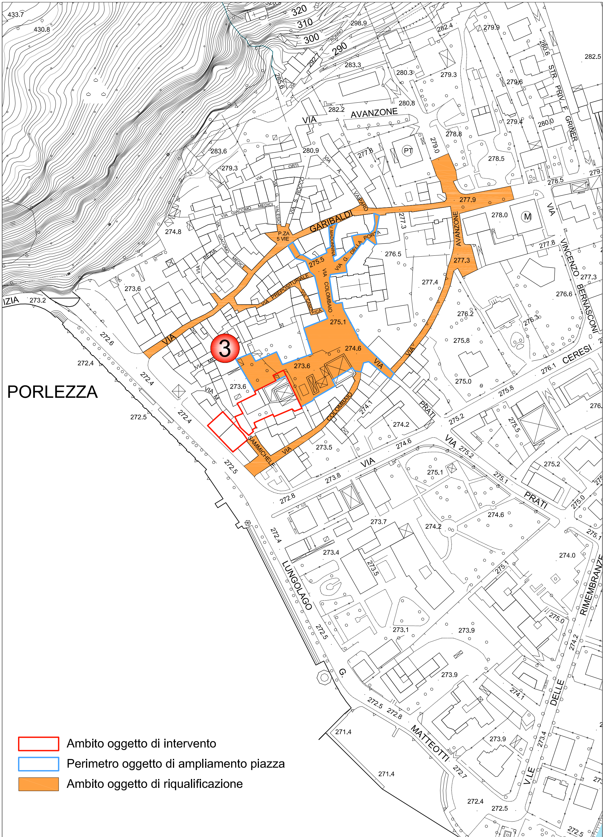
Stralcio aereofotogrammetrico - scala 1:2.000
