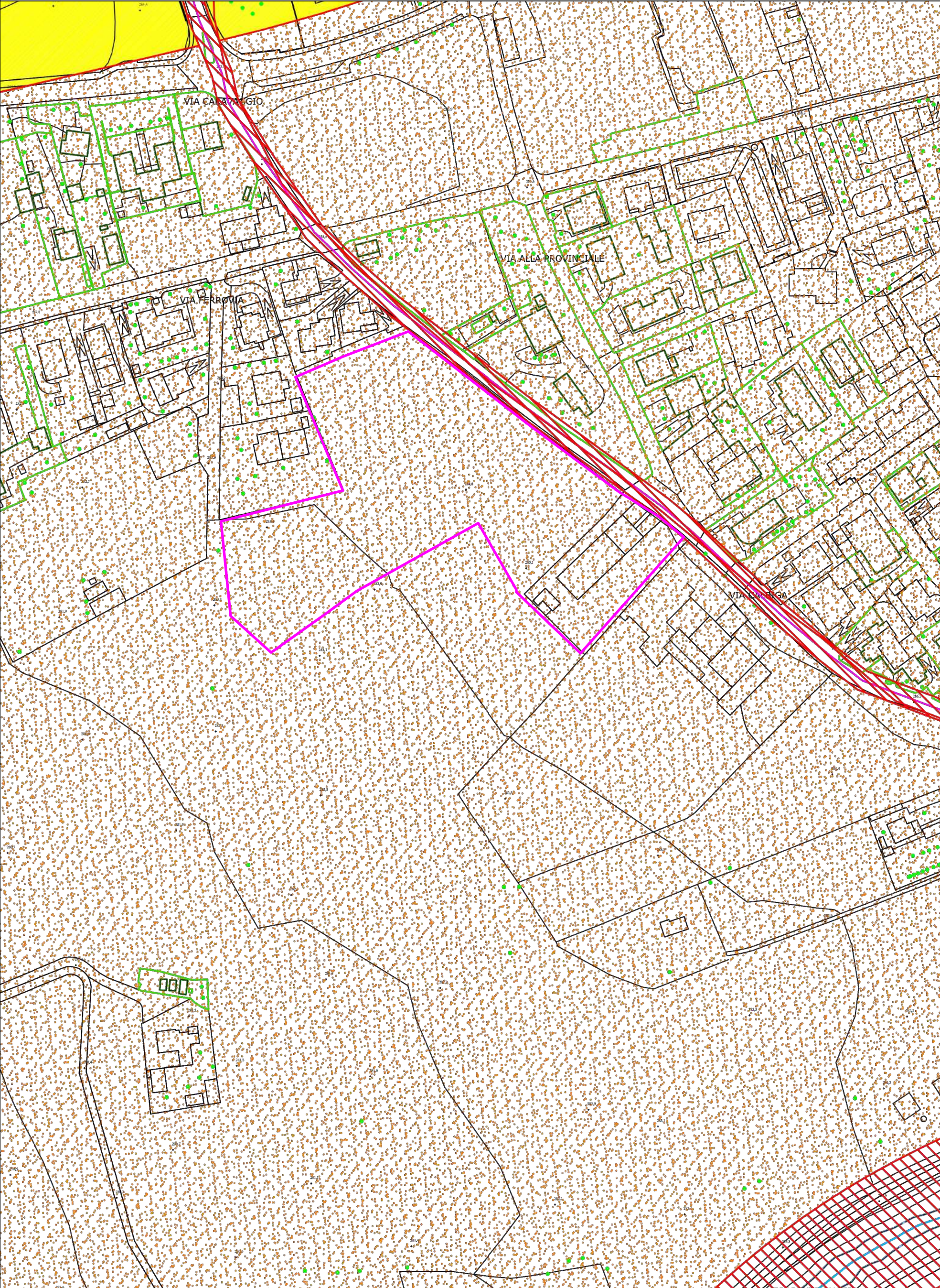
STUDIO GEOLOGICO
