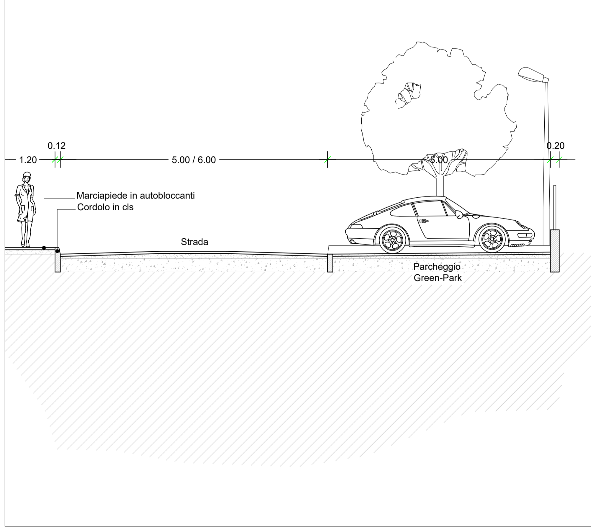
SEZIONE STRADALE TIPO scala 1:50
