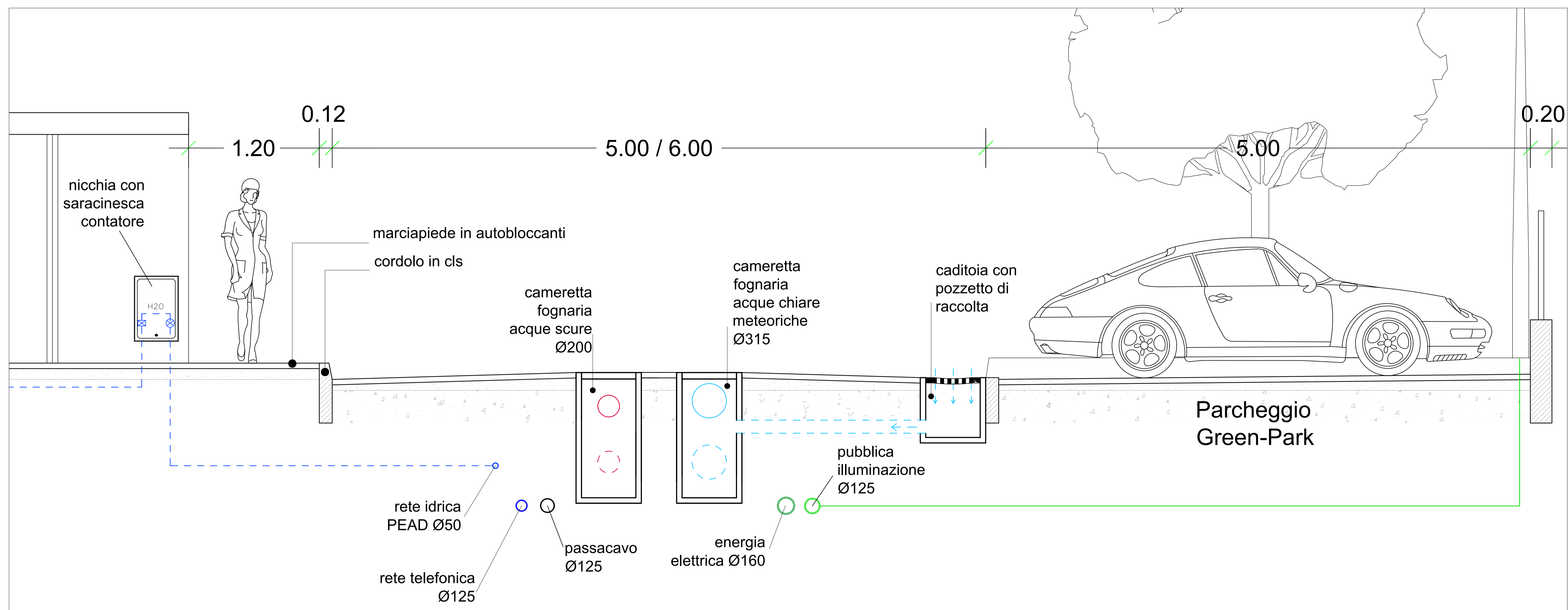
SEZIONE STRADALE TIPO CON SOTTOSERVIZI scala 1:20
